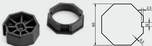
MS45 AP 01N 0B 00 Puleggia/corona per tubo ottagonale Ø60 Male/female adapter for Ø60 mm octagonal tube
