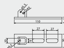
MS45 AS 06N 0G 00 Staffa di supporto regolabile - Zincato Bianco Adjustable support bracket - White Galvanized
