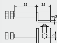
MS45 AS 04N 0G 00 Staffa di supporto regolabile a vite - Zincato Bianco Screw-adjustable support bracket - White Galvanized
